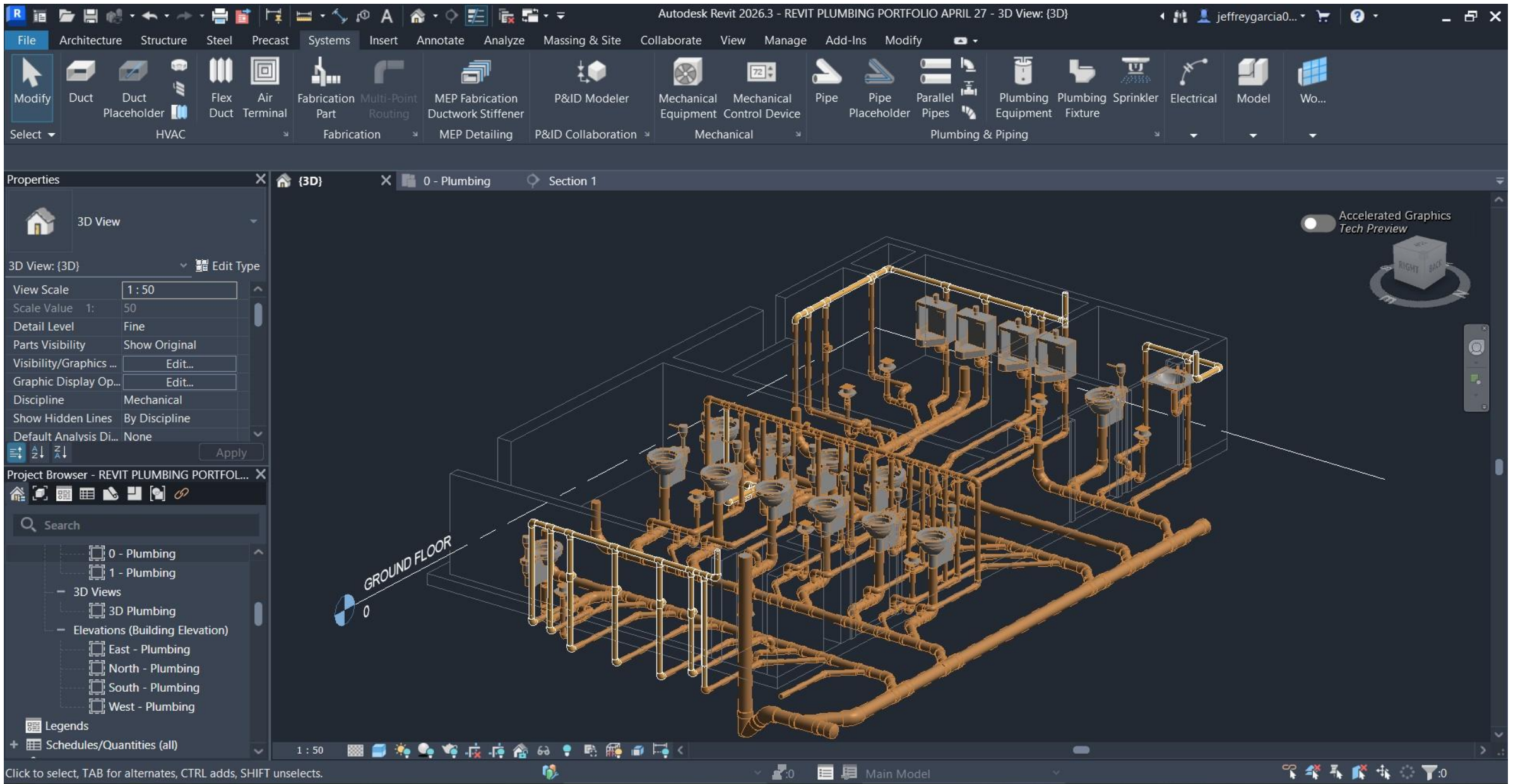
ROUGHING INS OF TOILET (REVIT MEP 2026)
